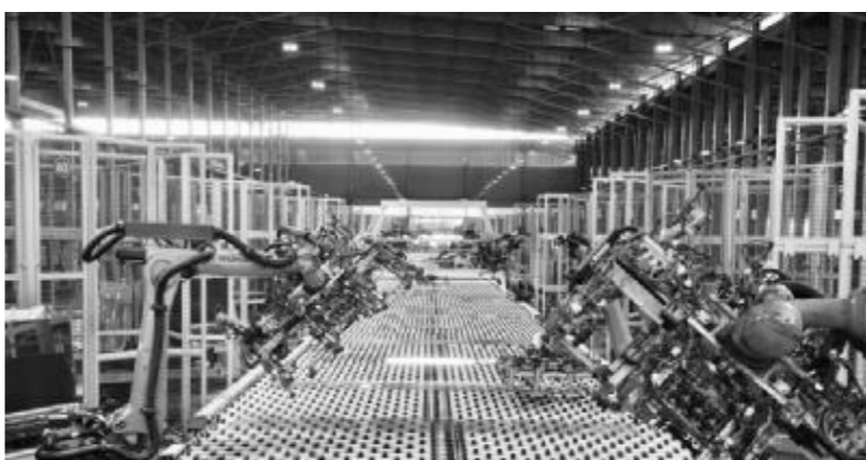
4月1日,在位于福建省福清市的福耀集团浮法玻璃生产线上,机械臂在抓取玻璃原片。
