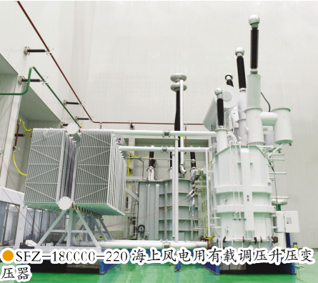
●SFZ-180000-220海上风电用有载调压升压变压器
