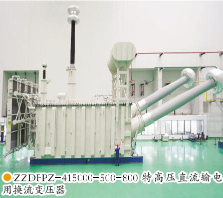
●ZZDFPZ-415000-500-800特高压直流输电用换流变压器
