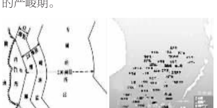
领海基线法示意图和南中国海实际被各国占领图例
