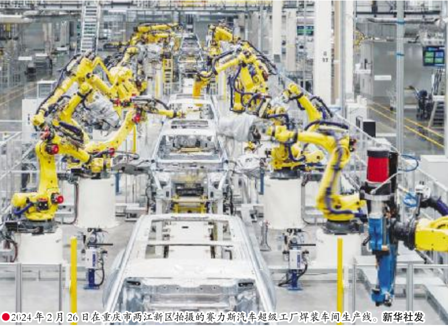
●2024 年 2 月 26 日在重庆市两江新区拍摄的赛力斯汽车超级工厂焊装车间生产线。新华社发
