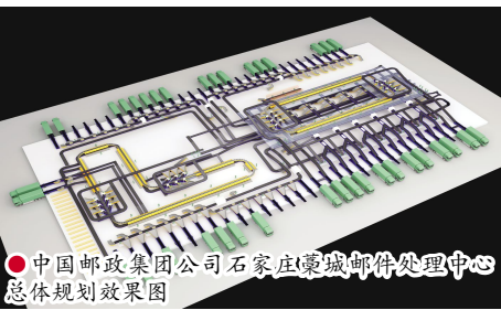
●中国邮政集团公司石家庄藁城邮件处理中心总体规划效果图
