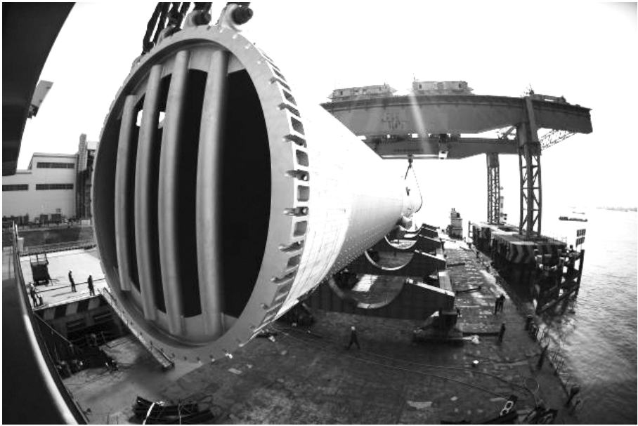
●在江苏镇江,260 万吨 / 年沸床床渣油锻焊加氢反应器正在进行吊装。 新华社记者 李响 摄
